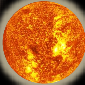
Enif
