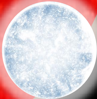
Deneb
