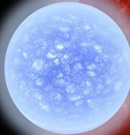
Pistol Star
