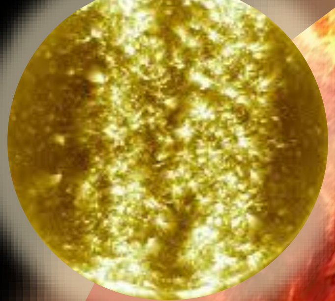
Rho Cassiopeiae
